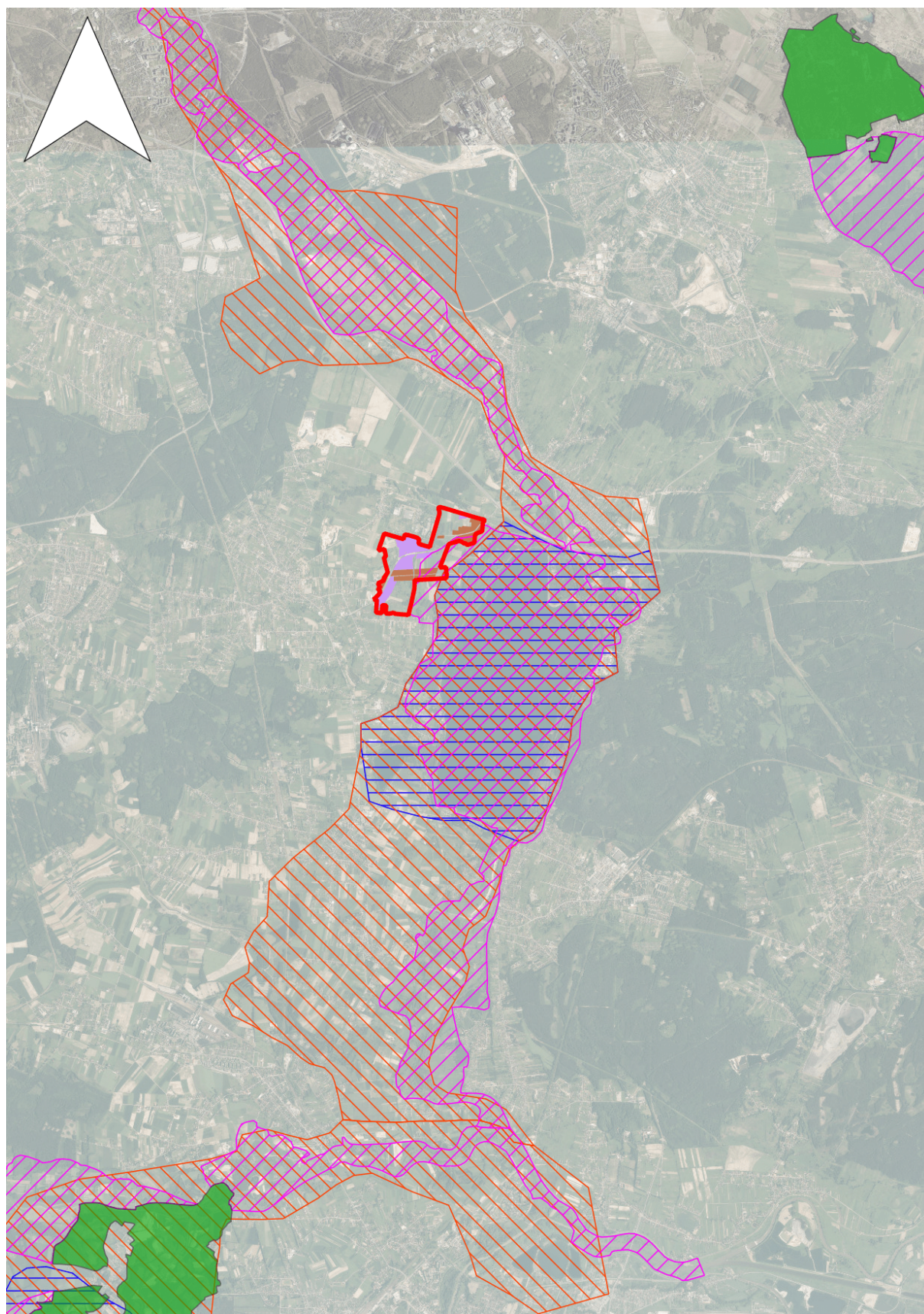
Rysunek 6 Położenie obszaru planu w relacji do korytarza spójności obszarów chronionych, korytarza omiotologicznego oraz przystanku dla ptaków, o których mowa w tekście prognozy (opracowanie własne na tle ortofotomapy, źródło mapy: www. geoportal.gov.pl ).
