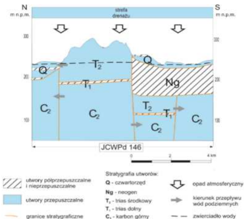
Rysunek 4 Schemat krążenia wód dla JCWPd nr 146 (źródło: https://www.pgi.gov.pl/dokumenty-pig-pib-all/psh/zadania-psh/jcwpd/jcwpd-140-159/4523-karta-informacyjna-jcwpd-nr-146/file.html )
